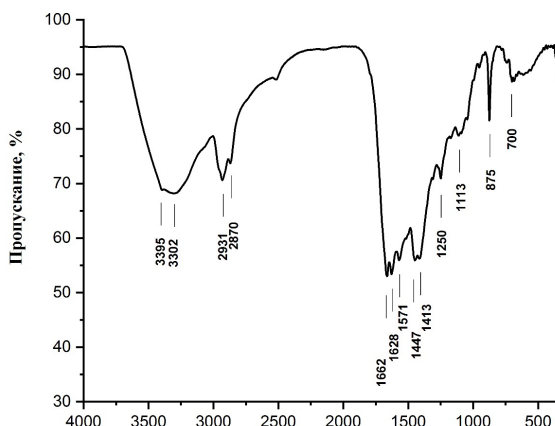
Рис. 2. ИК – спектр билирубинового камня (gall_3)
