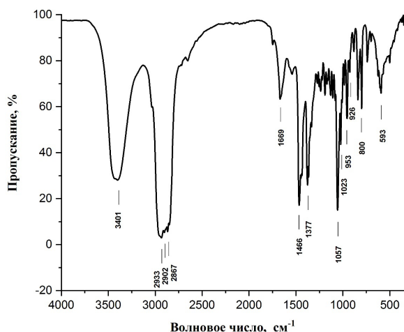
Рис. 1. ИК спектр холестеринного камня (gall_1)
